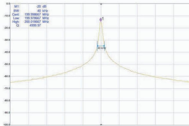
Lorentzian Linewidth (2kHz)
