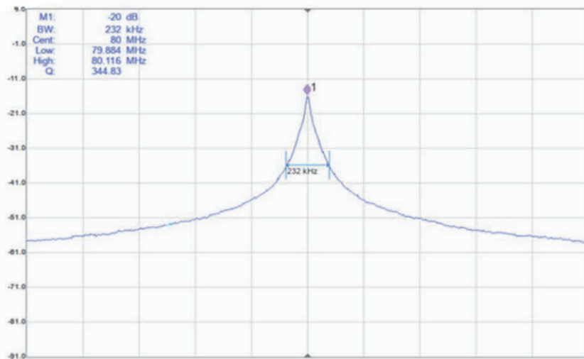
Lorentzian Linewidth (11.6kHz)
